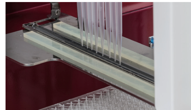
液だれ防止シャッター閉口時
