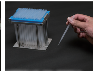
大容量チップ 10～1200μL
