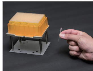
小容量チップ 1～100μL
